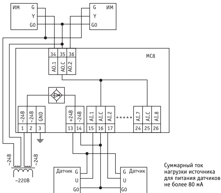
Рис. 9 – Пример подключения цепей питания датчиков 0 -10 В постоянного тока к контроллеру МС8.2х2хххх
