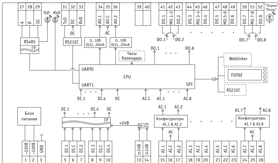
а) Функциональная схема контроллера МС8.1х1хххх (на ~220В)
