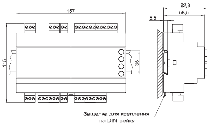
б) контроллер с разъемно-винтовыми клеммниками Рис. 7- Габаритные размеры и монтаж контроллеров
