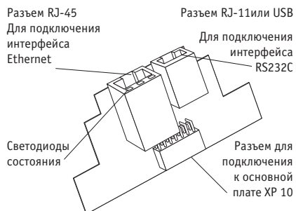
Рис.5 – Общий вид интерфейсного субмодуля WebLinker EM или WebLinker USB
