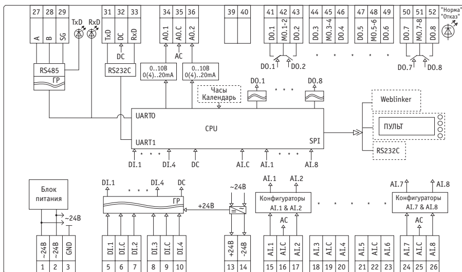
б) Функциональная схема контроллера МС8.2х2хххх (на ~24 В)
