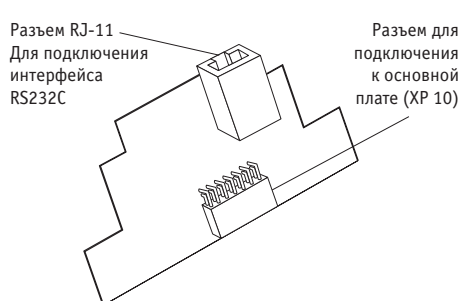
Рис.4 – Общий вид интерфейсного субмодуля RS232C или WebLinker Modem
