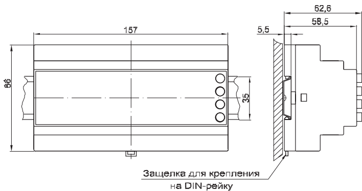
а) контроллер с винтовыми клеммниками
